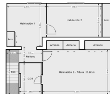
PRIMERA PLANTA
