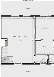
PLANTA BAJA
