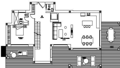
planta baja
