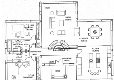
PLANTA BAJA
