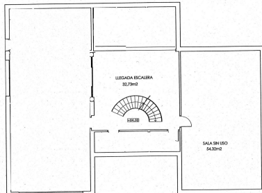
PLANTA SOTANO
