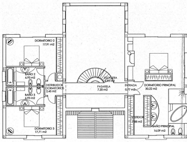
PLANTA ALTA
